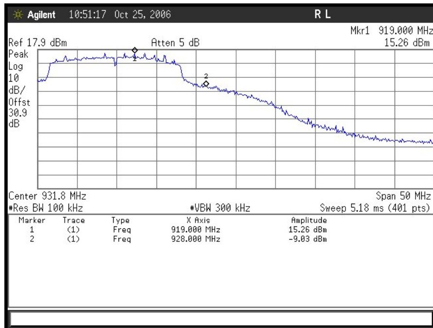
Plot 22. 802.11/b – 917MHz Upper Band Edge (OFDM 20MHz)
